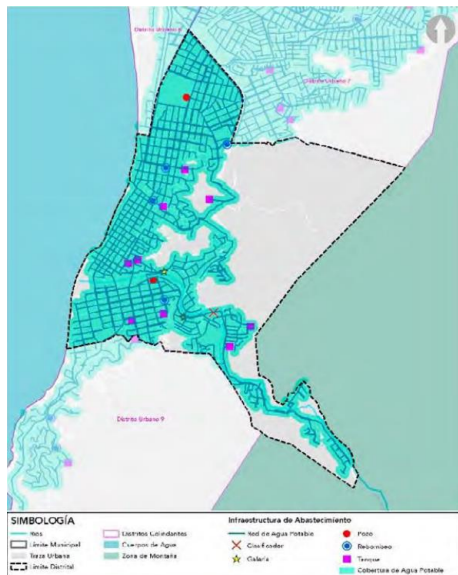
Figura 6. Redes de Agua Potable.
