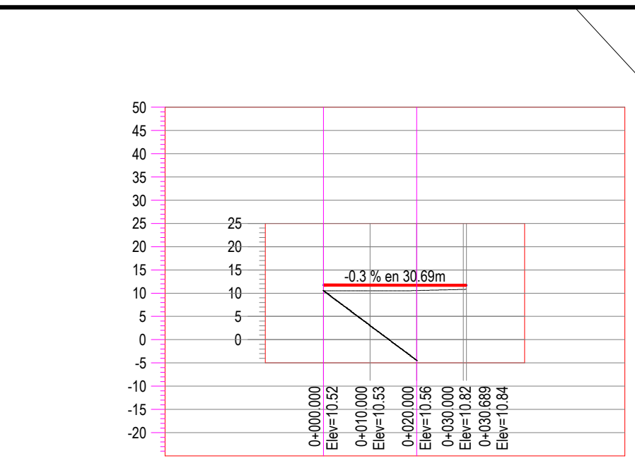
PERFIL 1 calle 02 ESCALA HORIZONTAL 1 : 1000 ESCALA VERTICAL 1 : 1000
